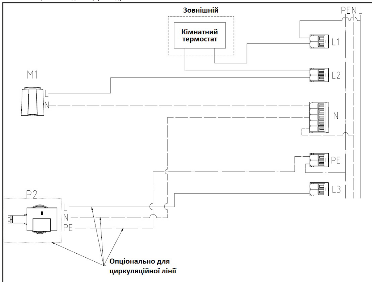
Схема електричних з'єднань (приклад)
