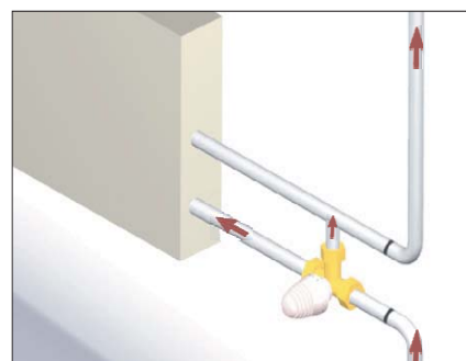
поток воды снизу вверх УТК - правый
