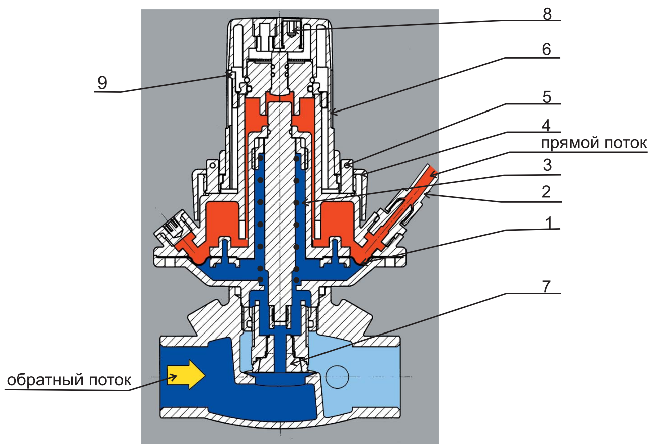
Рис. 4.21 Схема регулятора перепада давления 4007 в разрезе
