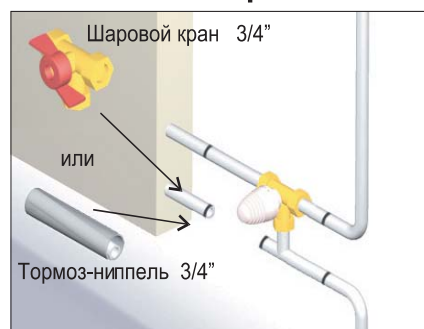
поток воды снизу вверх УТК - левый
