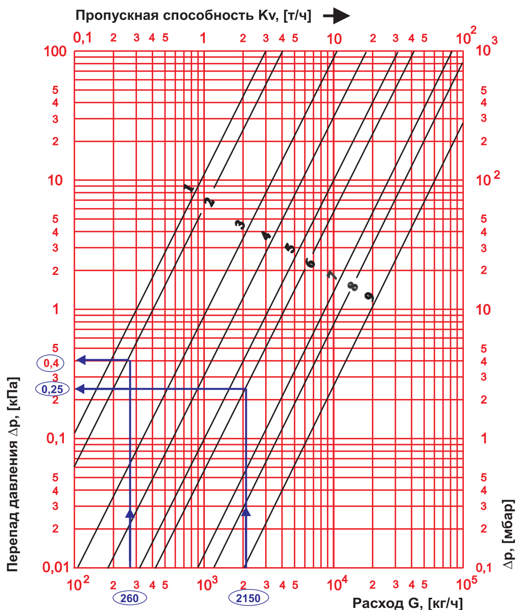
Рис. 4.12 Номограмма потерь давления запорного вентиля Штрёмаск (1 4115).
