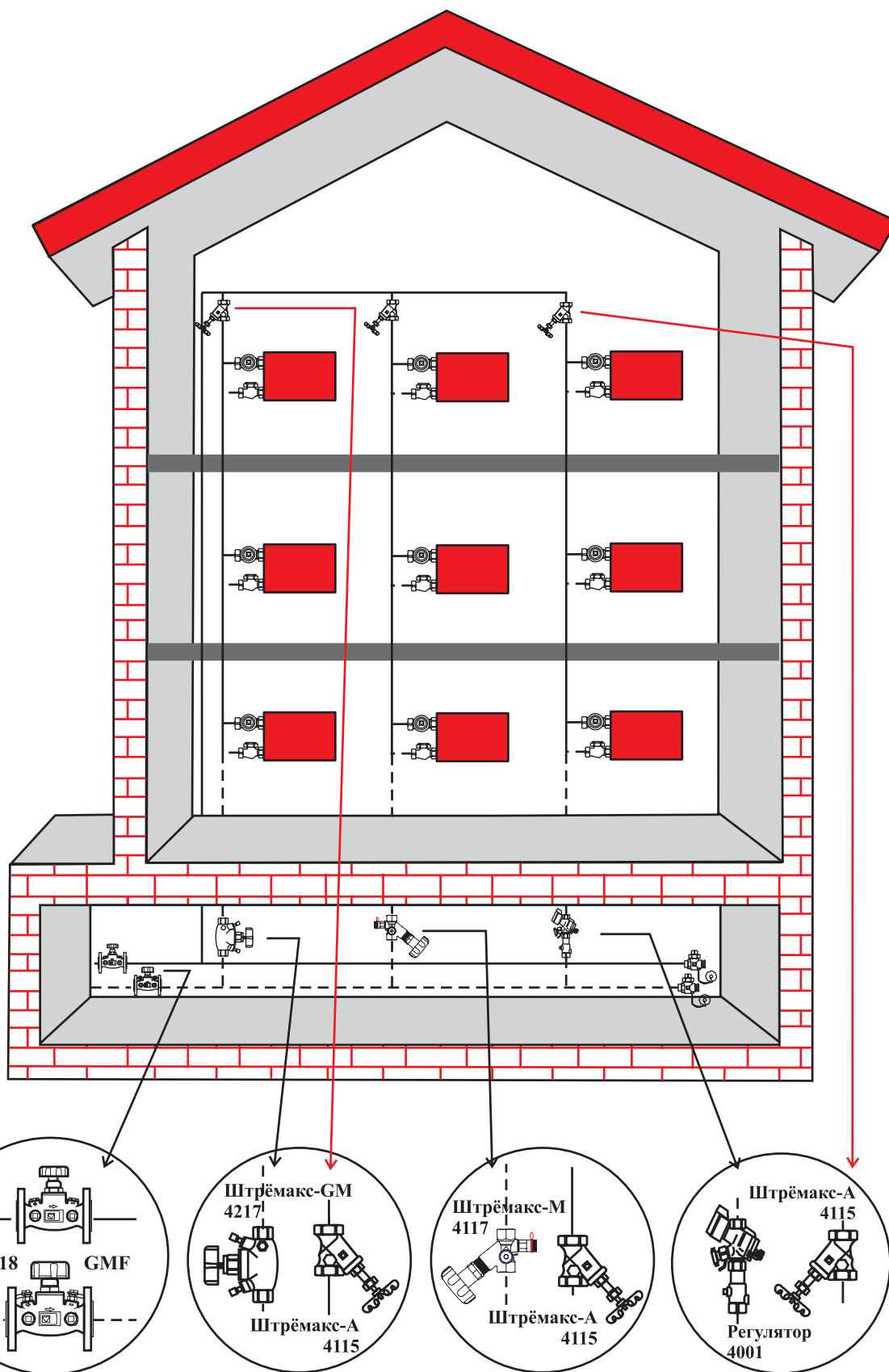
Рис. 4.3 Примеры установки балансировочной арматуры в однотрубной системе отопления.
